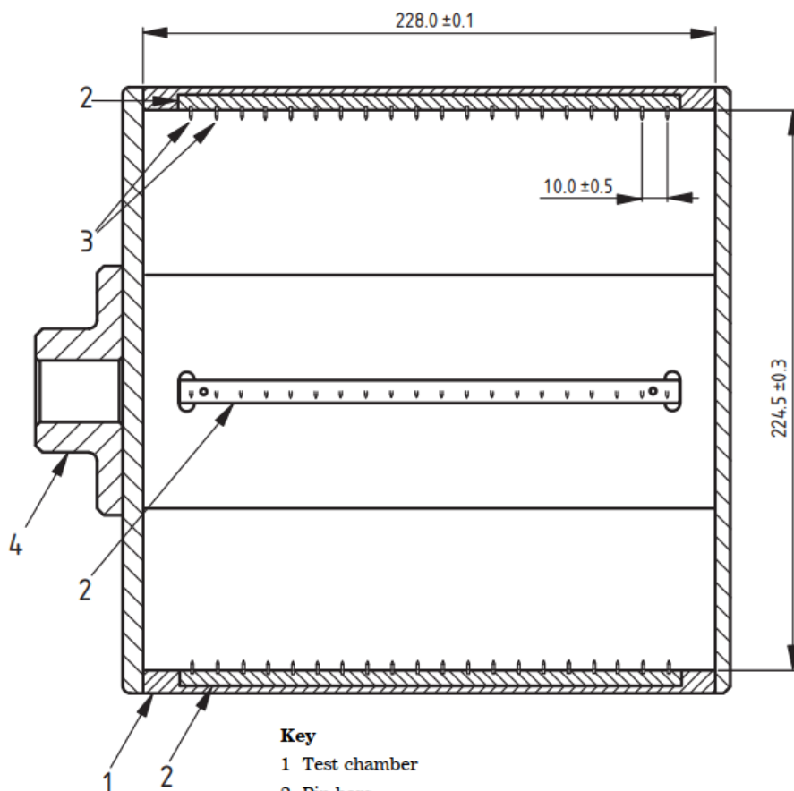
Mặt cắt ngang của hộp/ Sectional view of test chamber
